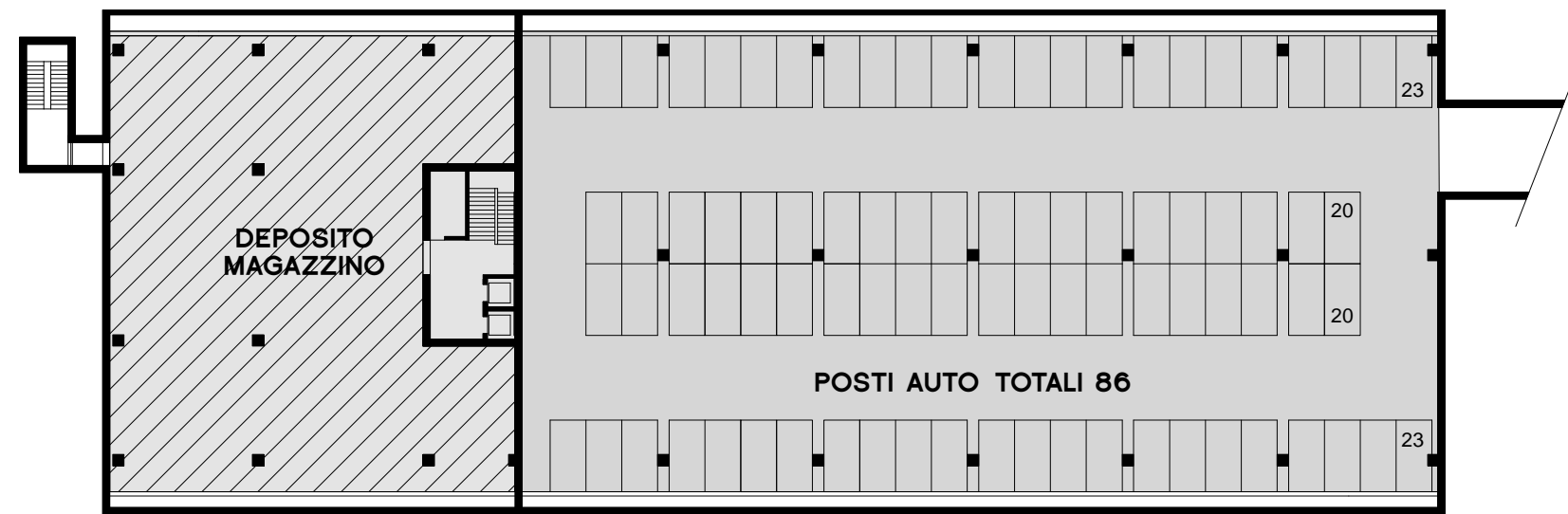
PIANTA LIVELLO -1
