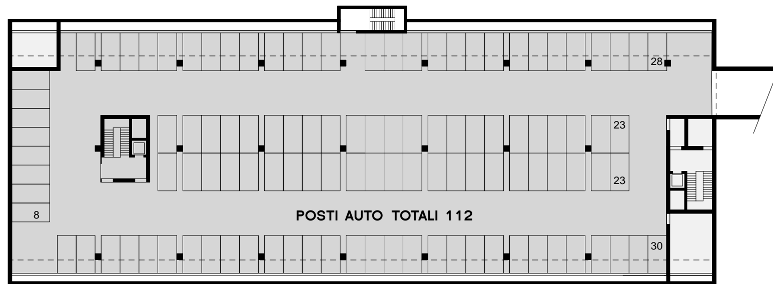
PIANTA LIVELLO -1
