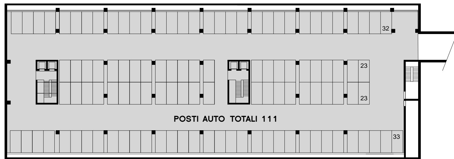
PIANTA LIVELLO -1
